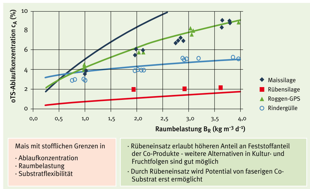
Abb. 23: Darstellung der oTS-Ablaufkonzentration bei verschiedener Raumbelastung unter Einsatz unterschiedlicher Substrate im Vergärungsfermenter einer Biogasanlage, verändert nach Mähnert, „Kinetik der Biogasproduktion aus nachwachsenden Rohstoffen und Gülle“, 2007
