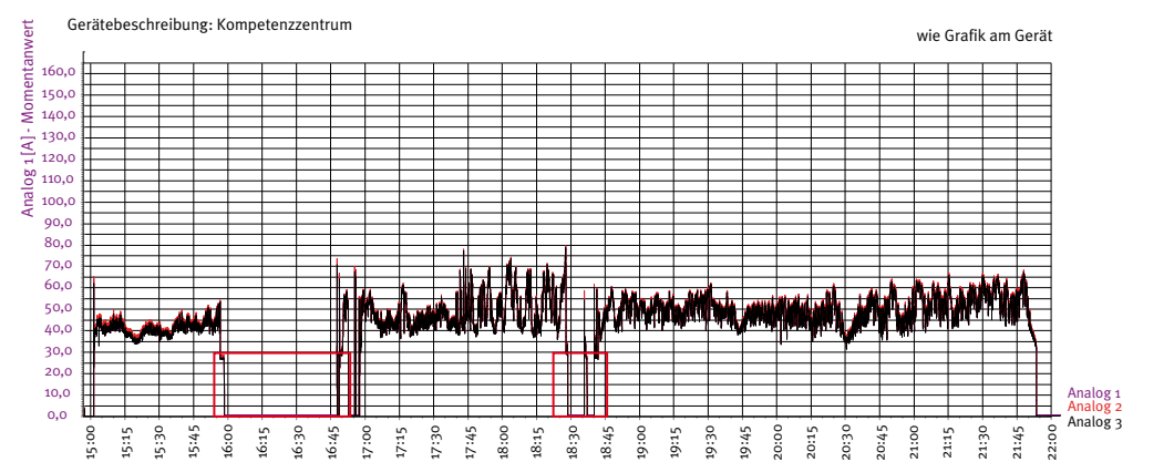
Abb.8: Verbrauchskurve des RZK 2010 (Zerkleinerer) im Auszug aus dem Strommessdiagramm (24.10.2012) – x-Achse (Zeit) und y-Achse (Ampere)
